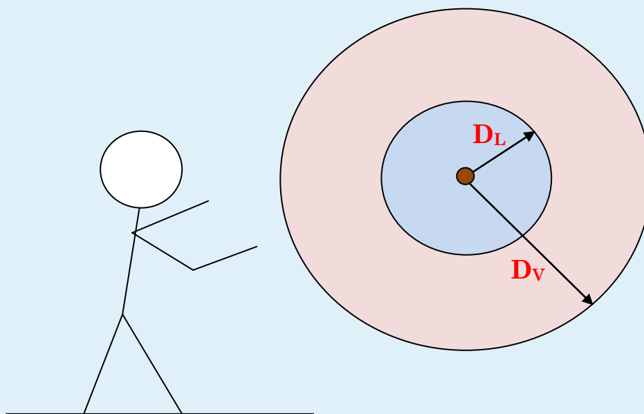
Figura n. 1 – distanze dalle parti attive (cerchio centrale in marrone) definite nella norma CEI 11-27, ai fini dell'individuazione del tipo di lavoro
